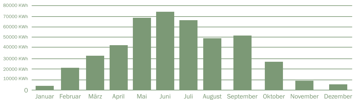
ERTRAGSVERLAUF DER PHOTOVOLTAIKANLAGE IM JAHR 2023 (IN SUMME RUND 500MWH SOLARSTROM)
