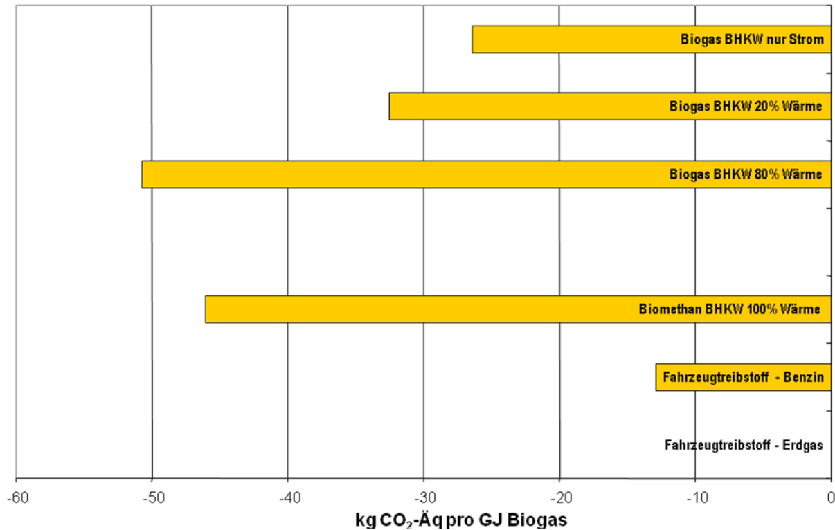
Abbildung 4.3.2.1: Bewertung verschiedener Optionen einer Biogasnutzung unter dem Klimaschutzaspekt im Vergleich zu Erdgas [IFEU, IE, Öko-Institut, 2007]
