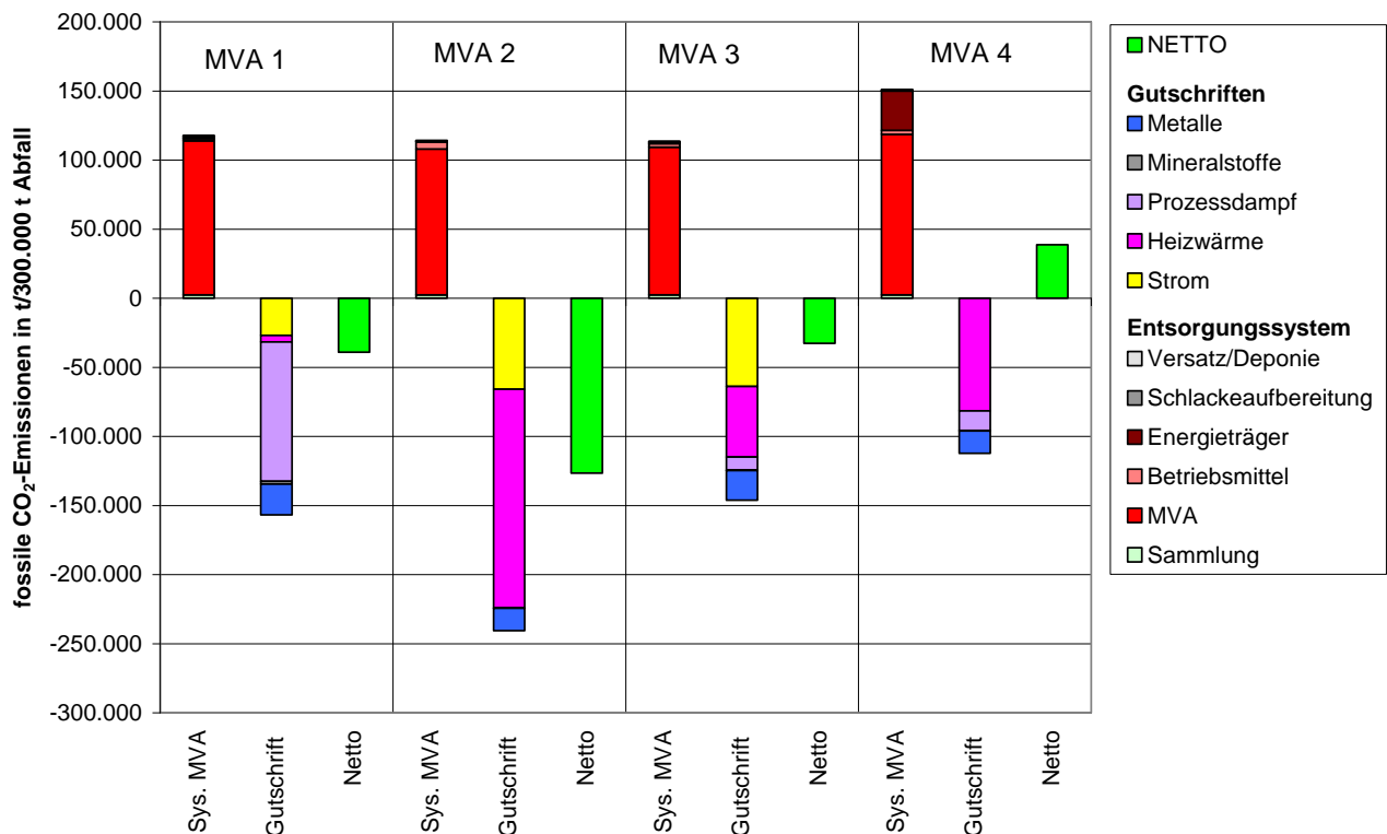
Abbildung 4.2.3: Analyse der CO 2 -Gesamtbilanz von vier energetischen Konzepten; Netto = \Sigma System MVA – \Sigma Gutschrift [IFEU, 2007]
