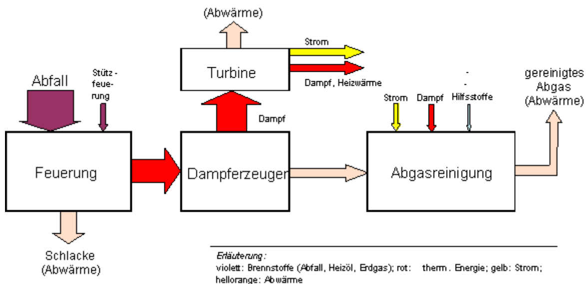
Abbildung 4.2.1: Stark vereinfachtes Schema des Energiestroms einer thermischen Restabfallbehandlungsanlage [IFEU, 2007]
